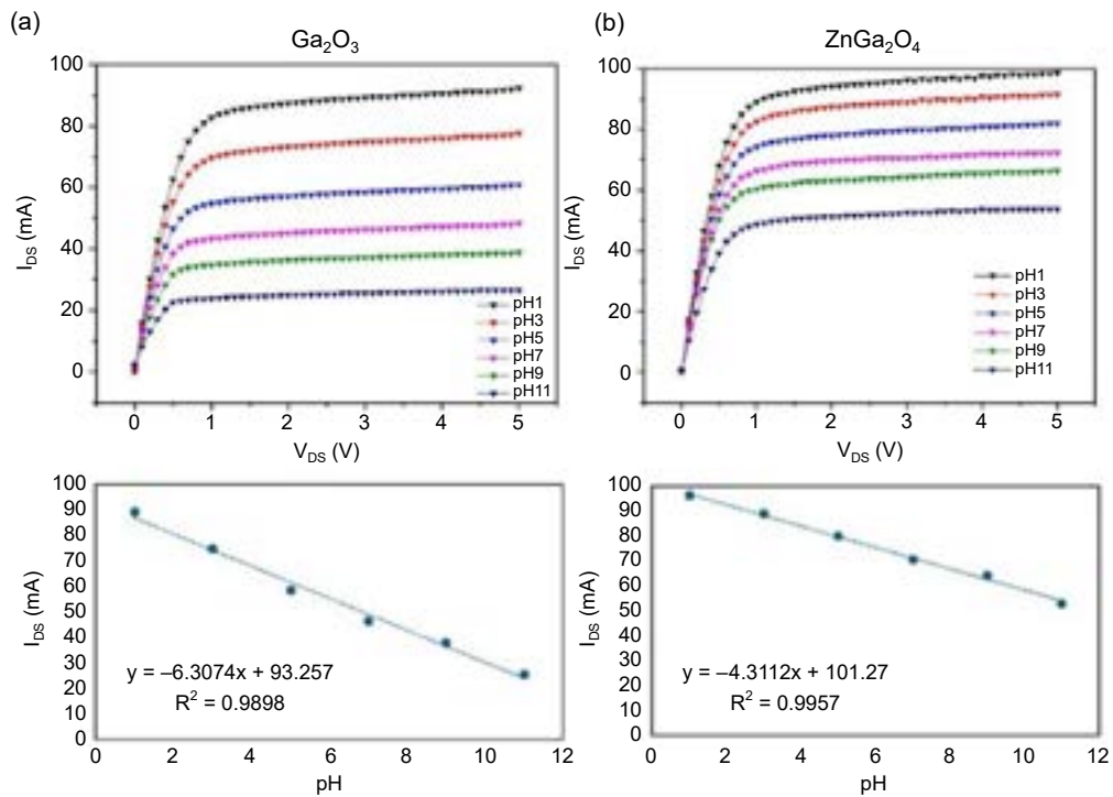
圖 9. (a) Ga_2O_3 與 (b) ZnGa_2O_4 EGFET 感測器在不同濃度 pH 溶液中的飽和值感測曲線與劑量依賴特性之線性分析。
