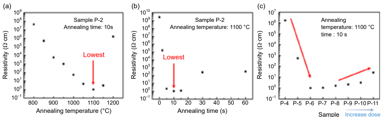
圖 4. Sample P-2 (a) 不同退火溫度 (b) 不同退火時間 與電阻率之關係圖 (c) 不同 P 離子佈植劑量與電阻率之關係圖 (Sample P-4 至 P-11)。
