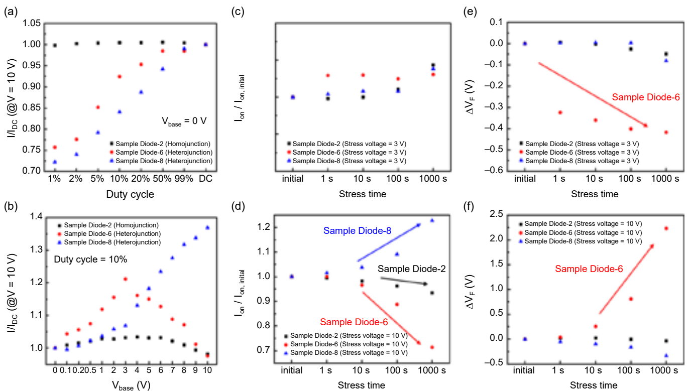
圖 12. (a) 不同 Duty cycle、(b) 不同 V_{base} 脈衝量測下開態電流與 DC 模式下開態電流之比值之整理圖、元件在 (c) V_{stress} = 3 V 、(d) V_{stress} = 10 V 下之 Stress 時間與開態電流的關係圖、元件在 (e) V_{stress} = 3 V 、(f) V_{stress} = 10 V 下之 Stress 時間與開啟電壓的關係圖。
